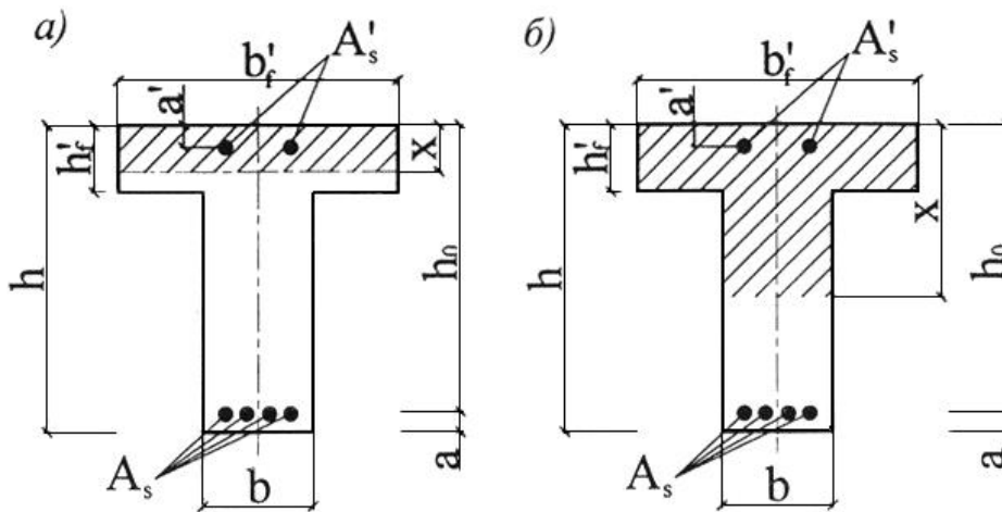
Рисунок 7.3 - Положение границы сжатой зоны в сечении изгибаемого железобетонного элемента
