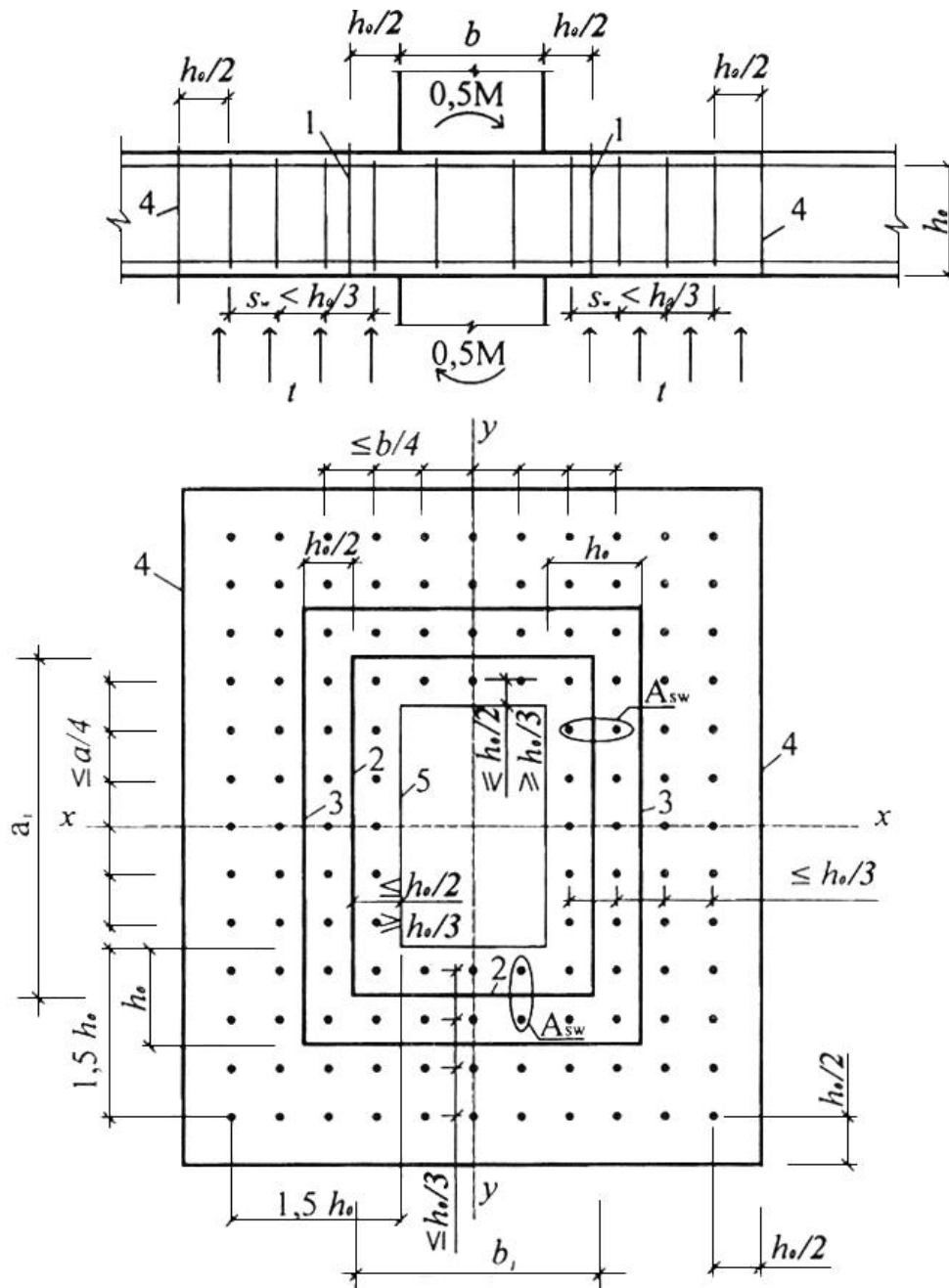
Рисунок 7.11 - Схема для расчета на продавливание железобетонной плиты с вертикальной равномерно распределенной поперечной арматурой при температурном воздействии снизу плиты
