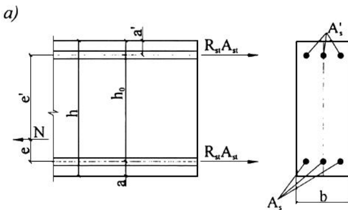
Рисунок 7.5 - Схема усилий и эпюра напряжений в сечении, нормальном к продольной оси внецентренно растянутого железобетонного элемента, при расчете его по прочности
