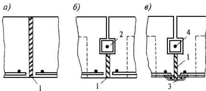
Рисунок 9.2 - Температурные швы в конструкциях из жаростойкого бетона
