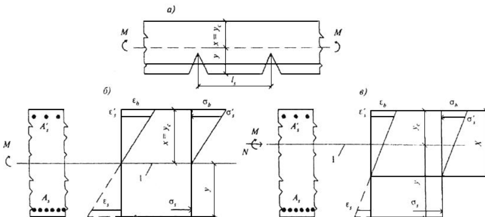
Рисунок 8.2 - Схема напряжений и деформаций в сечении с трещиной при действии изгибающего момента, изгибающего момента и продольной силы
