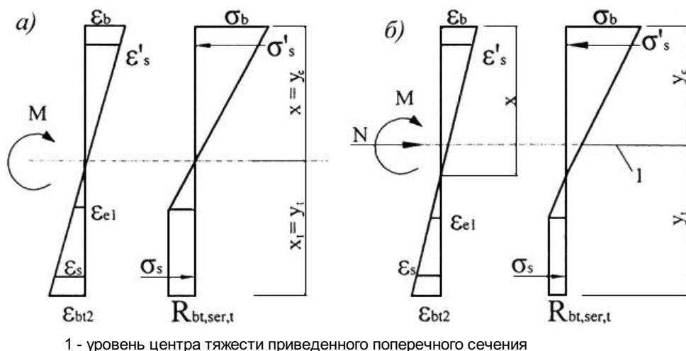
Рисунок 8.1 - Схема напряженно-деформированного состояния сечения элемента при проверке образования трещин при действии изгибающего момента (а), изгибающего момента и продольной силы (б)
