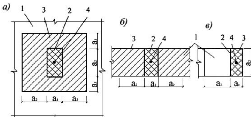
Рисунок 7.8 - Схемы для расчета элементов на местное сжатие при расположении местной нагрузки
