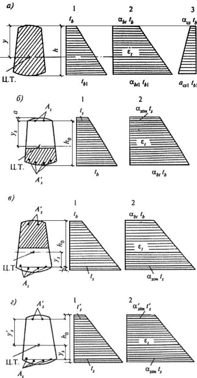
Рисунок 6.3 - Схемы распределения температур, деформаций от неравномерного нагрева и остывания при прямолинейном изменении температур по высоте сечения элементов
