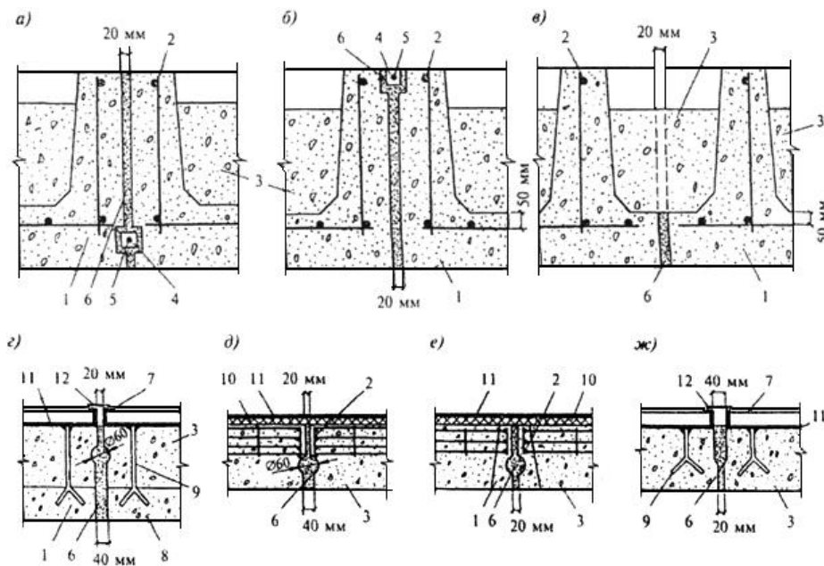
Рисунок 9.1 - Стыки элементов сборных конструкций из жаростойкого бетона
